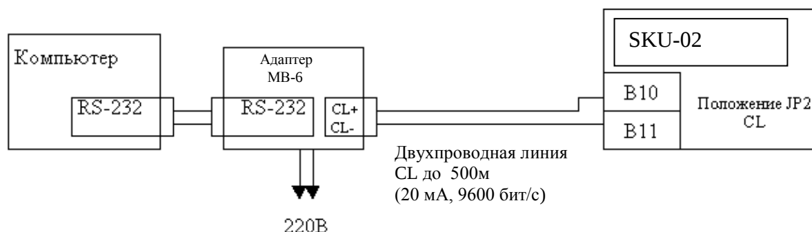
Рисунок К.3. Схема подключения компьютера или модема при помощи адаптера MB-6. Длина линии связи до 500 метров (до 9600 бит/с, 20мА). Интерфейс счетчика “Токовая петля” (CL).
