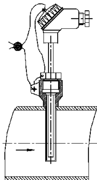
Рис. И.2. Схема монтажа термопреобразователя с монтажной головкой на трубопроводе с защитной гильзой (только для трубопровода DN > 50 ).
