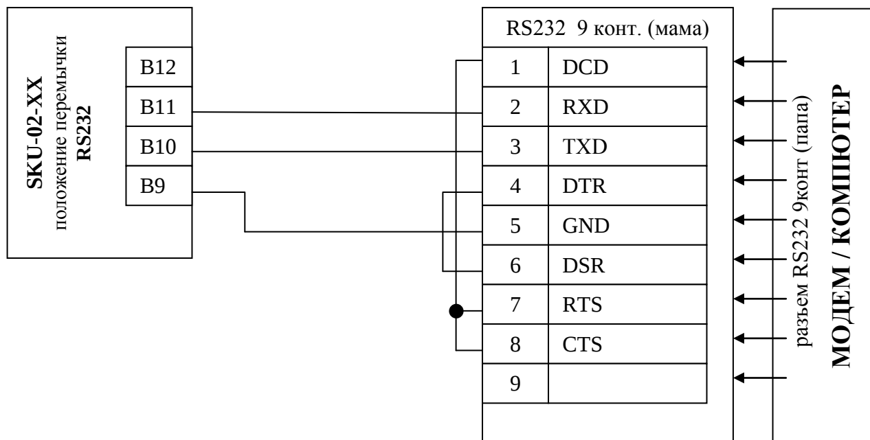
Рисунок К.2. Схема подключения счетчика по интерфейсу RS 232.
