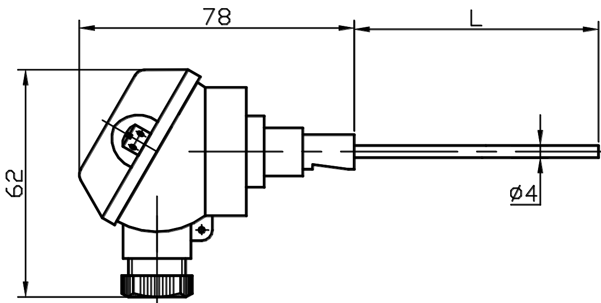
Рис. И.3. Габаритные размеры термопреобразователя сопротивления КТСП-Н. L - Длина монтажной части от 80 до 250 мм.
