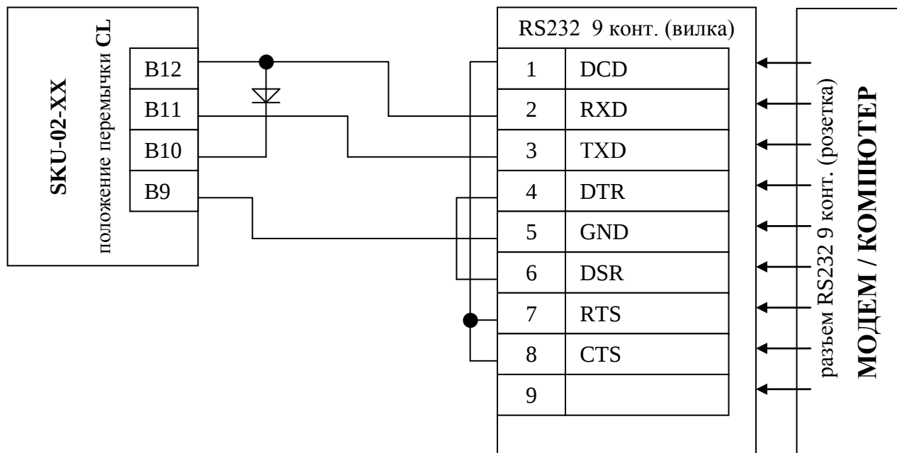
Рисунок К.1. Схема подключения счетчика по интерфейсу «Токовая петля (CL)». Диод – любой маломощный (например, КД 503).
