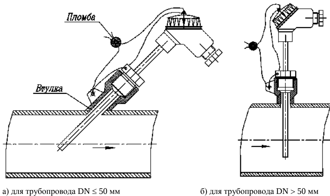
Рис. И.1. Схема монтажа термопреобразователя на трубопроводе без защитной гильзы
