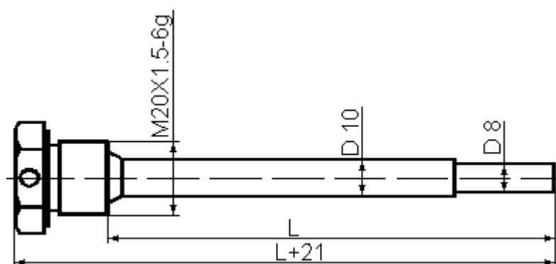
Рис. И.4. Габаритные размеры гильзы с креплением термопреобразователя винтом с отверстием под пломбировку L - Длина монтажной части от 80 до 250 мм.
